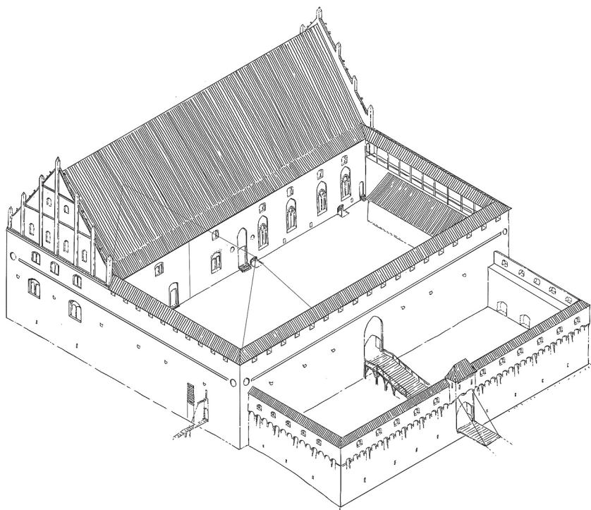
Ryc. 13. Próba rekonstrukcji zamku w Słońsku pod koniec XV w. Wykonał K. Wroński
