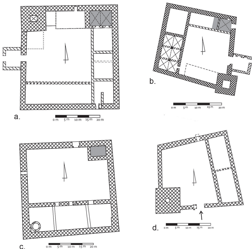
Ryc. 6. Rzut poziomy zamków w Swobnicy (a), Łagowie (b), Starym Drawsku (c) i Pęzinie (d). Kolorem szarym oznaczono przypuszczalną lokalizację kaplic. Wykonał K. Wroński
