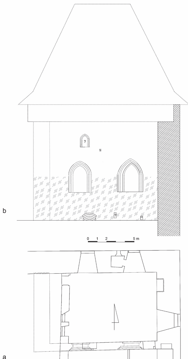
Ryc. 11. Rekonstrukcja elewacji południowej kaplicy na zamku w Swobnicy. Wykonał K. Wroński
